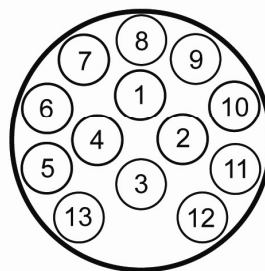
DIN/ISO 11446 13-pol
